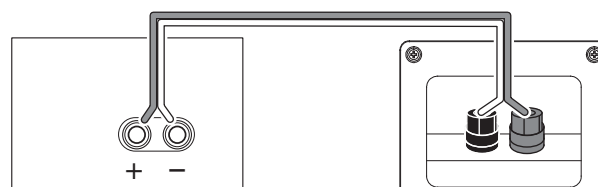
Приемник или усилитель (показан один канал)
