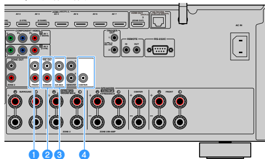
Аппарат (вид сзади)
