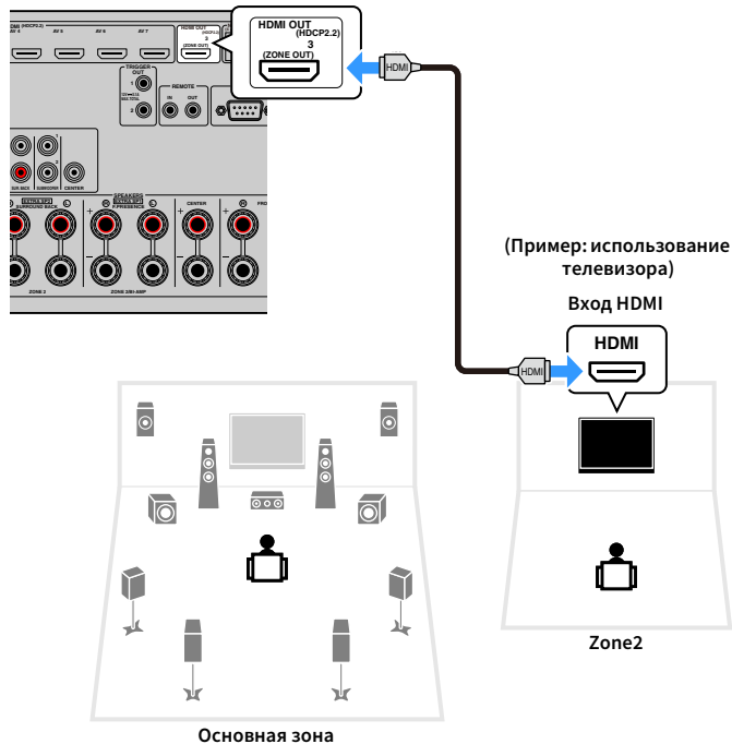
Аппарат (вид сзади) Гнездо HDMI OUT 3 (ZONE OUT)
