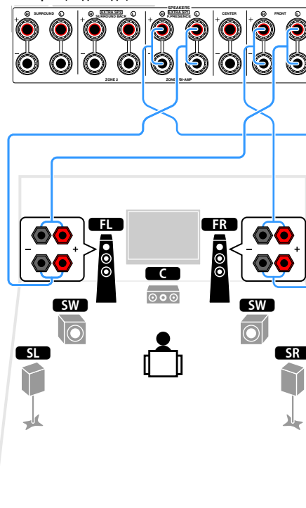
Аппарат (вид сзади)
