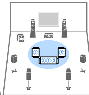
Многопозиционное измерение (5 положений прослушивания)
